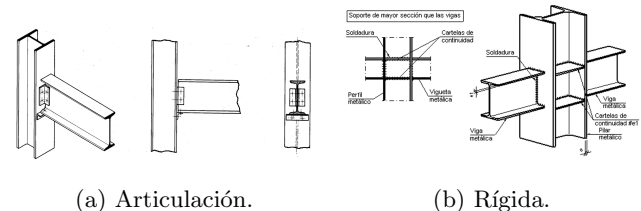
Figura 2.17: Nudos.
