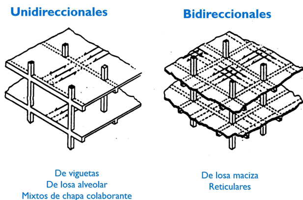
Figura 2.28: Forjados. Tipologías
