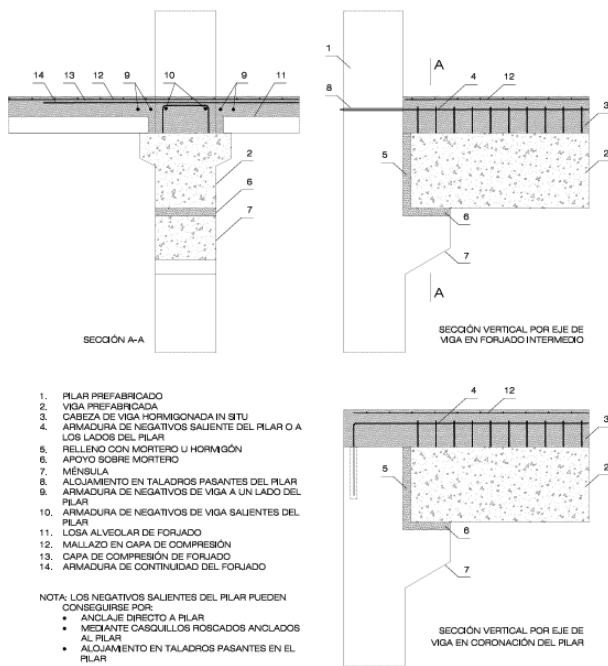
Figura 2.32: Forjados. Apoyos
