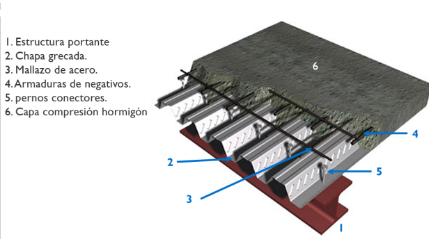
Figura 2.33: Forjado de chapa colaborante.
