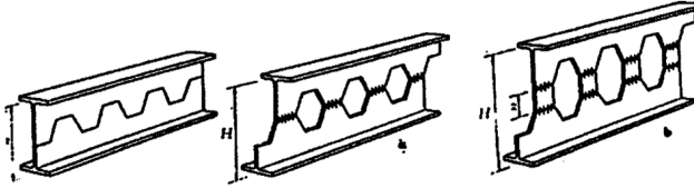
Figura 2.15: Vigas Aligeradas o Vigas Boyd
