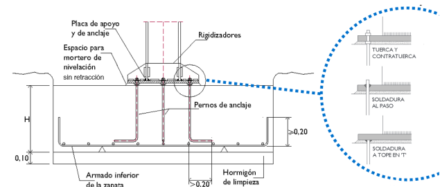
Figura 2.18: Nudo Cimentación.
