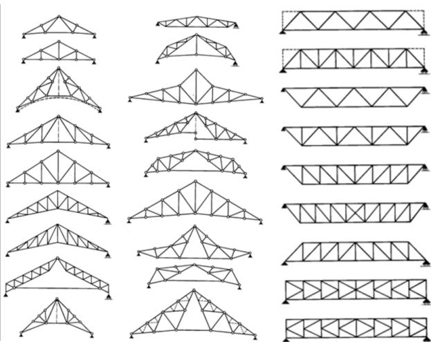
Figura 2.16: Cercas y celosías
