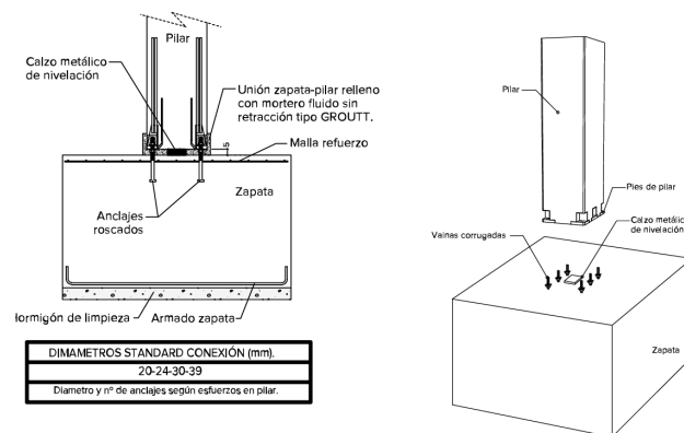
Figura 2.27: Empotramiento con anclajes roscados.
